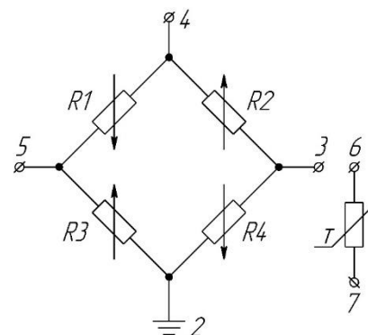
Замкнутый мост
