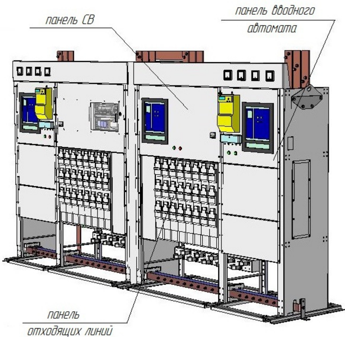
Рис. 6 Внешний вид НКУ-Орб11Б
